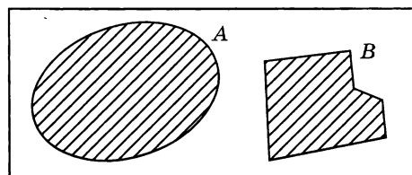
A и B несовместны
