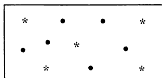
Из них: N(A) благоприятствующих событию A
